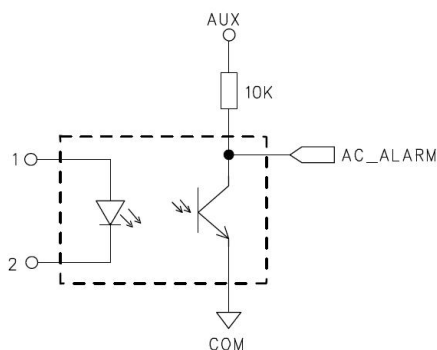
AC_ALARM 信号连接方式
