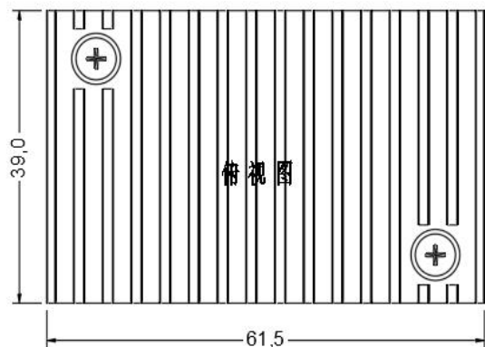
标准型+散热器 61.5*39.0*27.7mm
