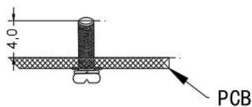
标准型 60.4*39.0*12.7mm
