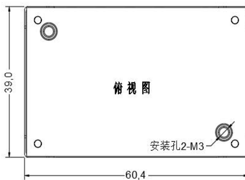
标准型 60.4*39.0*12.7mm
