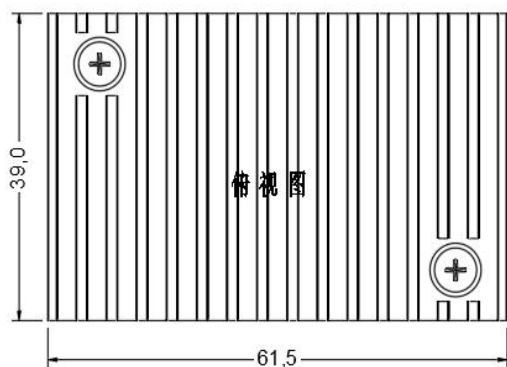
标准型+散热器 61.5*39.0*27.7mm
