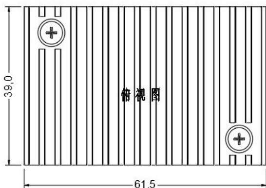
标准型+散热器
