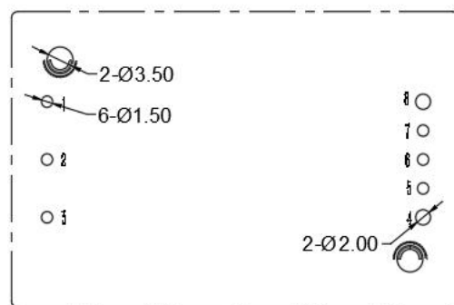
推荐PCB开槽尺寸
