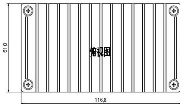
标准型+散热器
