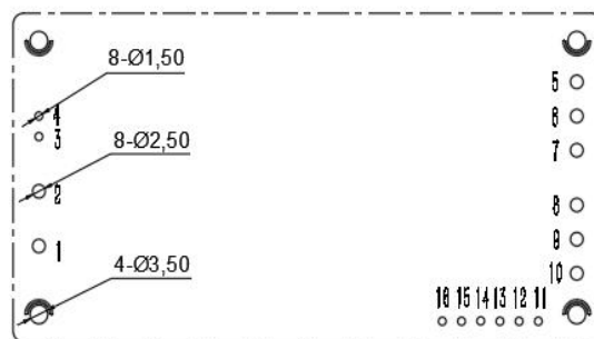
推荐PCB开槽尺寸
