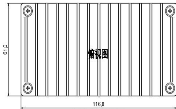
标准型+散热器
