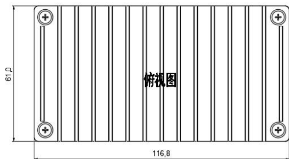
标准型+散热器 116.8*61.0*32.7mm
