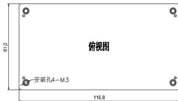
标准型 116.8*61.0*12.7mm
