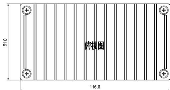
标准型+散热器 116.8*61.0*32.7mm
