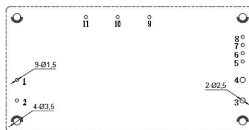
推荐PCB开槽尺寸
