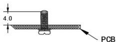
标准型 61.0*57.9*12.7mm
