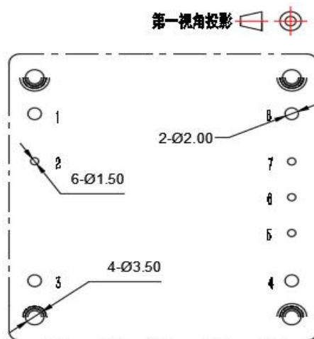
推荐PCB开槽尺寸
