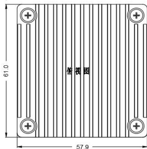
标准型+散热器 61.0*57.9*27.7mm
