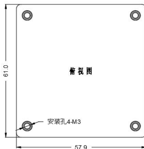
标准型 61.0*57.9*12.7mm
