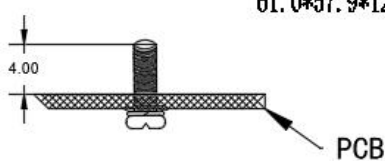
标准型 61.0*57.9*12.7mm
