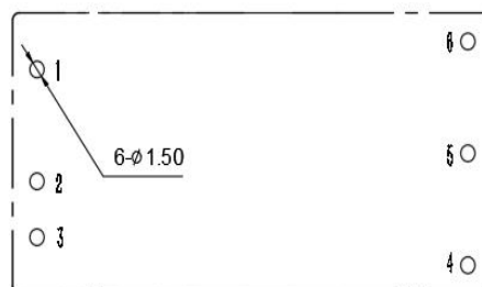
推荐PCB开槽尺寸
